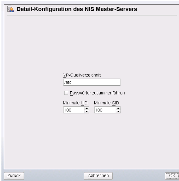
Abbildung 19.3 Ändern des Verzeichnisses und Synchronisieren von Dateien für einen NIS-Server
