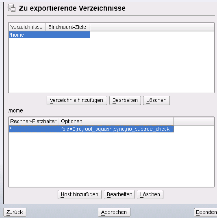
Abbildung 21.3 Konfigurieren eines NFS-Servers mit YaST
