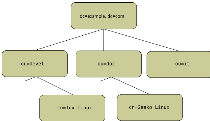
Abbildung 20.1 Struktur eines LDAP-Verzeichnisses
