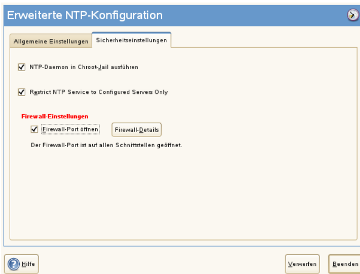
Abbildung 18.3 Erweiterte NTP-Konfiguration: Sicherheitseinstellungen
