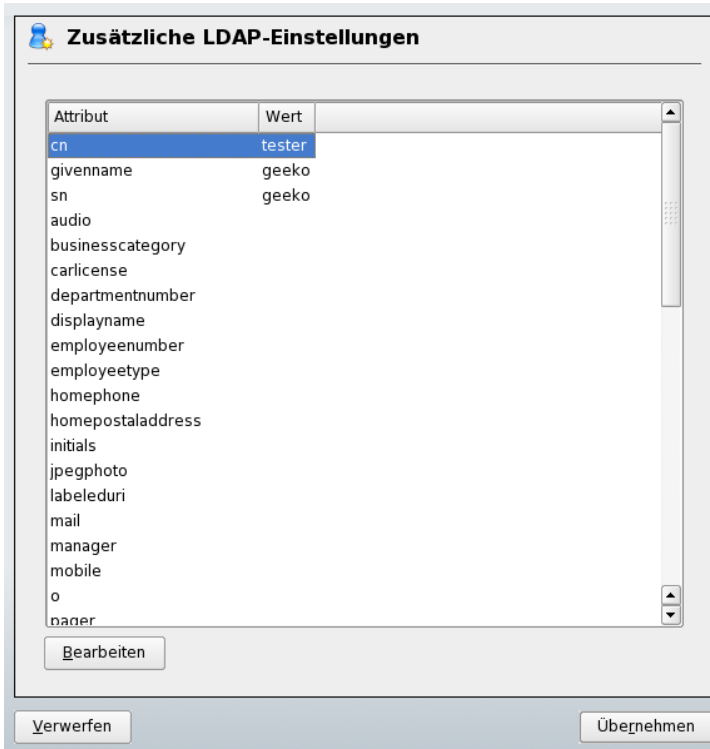
Abbildung 20.7 YaST: Zusätzliche LDAP-Einstellungen
