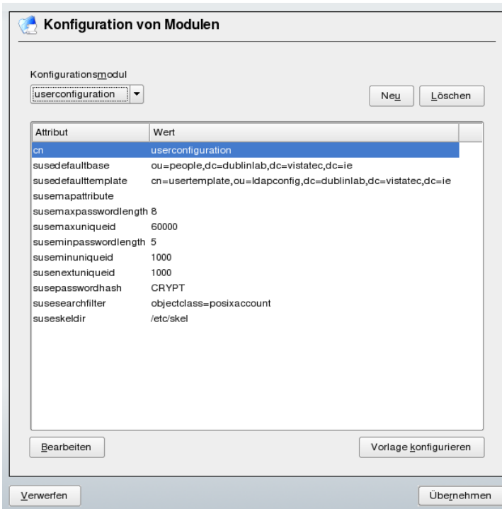
Abbildung 20.5 YaST: Modulkonfiguration
