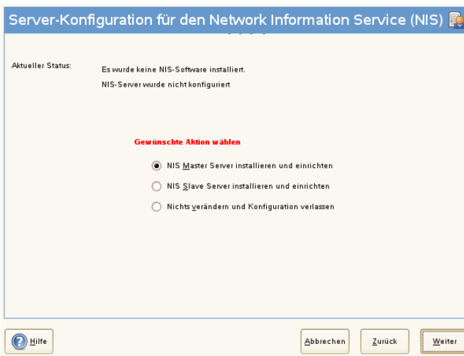
Abbildung 19.1 NIS-Serverkonfiguration
