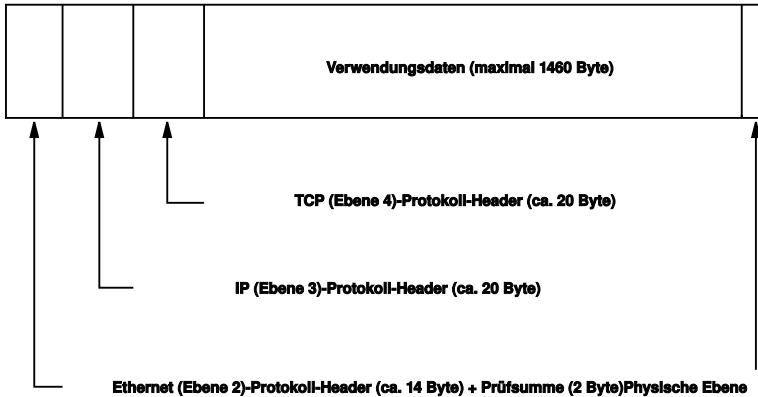
Abbildung 14.2 TCP/IP-Ethernet-Paket
