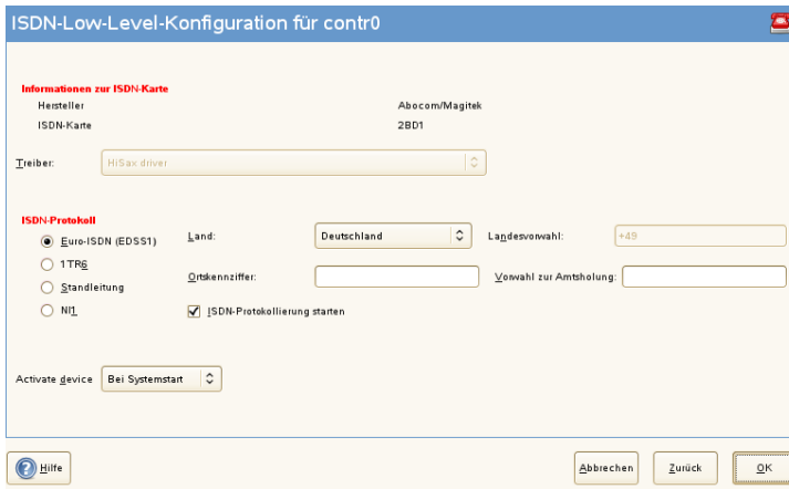
Abbildung 14.5 ISDN-Konfiguration
