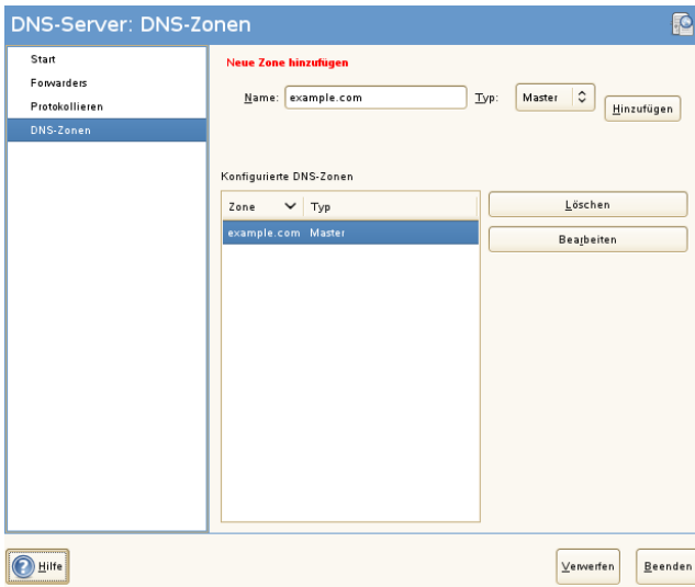
Abbildung 16.2 DNS-Server-Installation: DNS-Zonen
