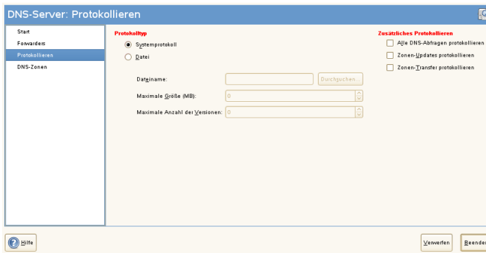
Abbildung 16.4 DNS-Server: Protokollieren
