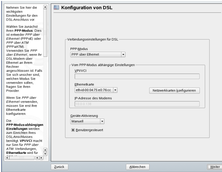
Abbildung 14.7 DSL-Konfiguration
