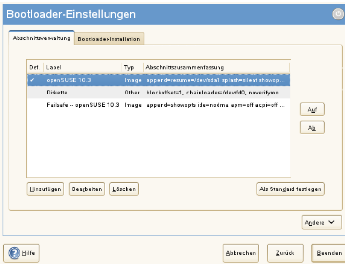
Abbildung 9.1 Bootloader-Einstellungen
