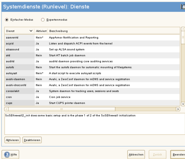
Abbildung 8.1 Systemdienste (Runlevel)
