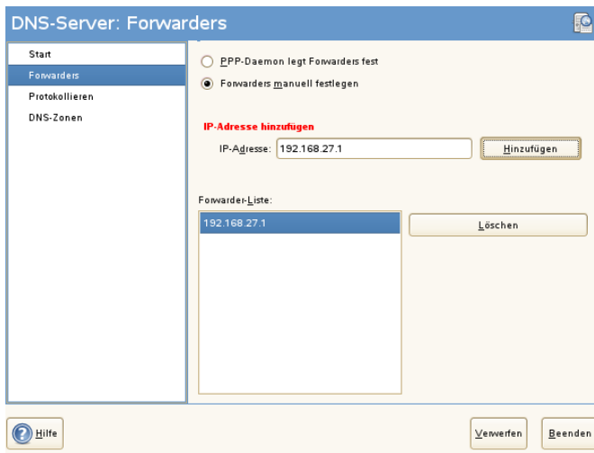
Abbildung 16.1 DNS-Server-Installation: Forwarder-Einstellungen
