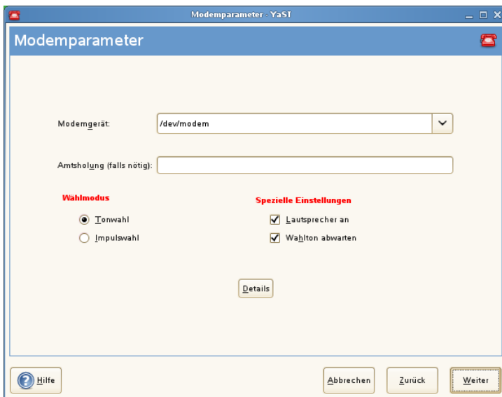
Abbildung 14.4 Modemkonfiguration
