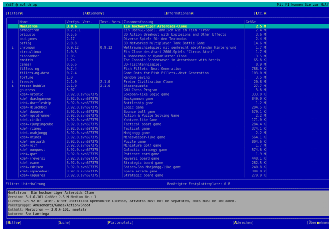
Abbildung 4.2 Das Software-Installationsmodul
