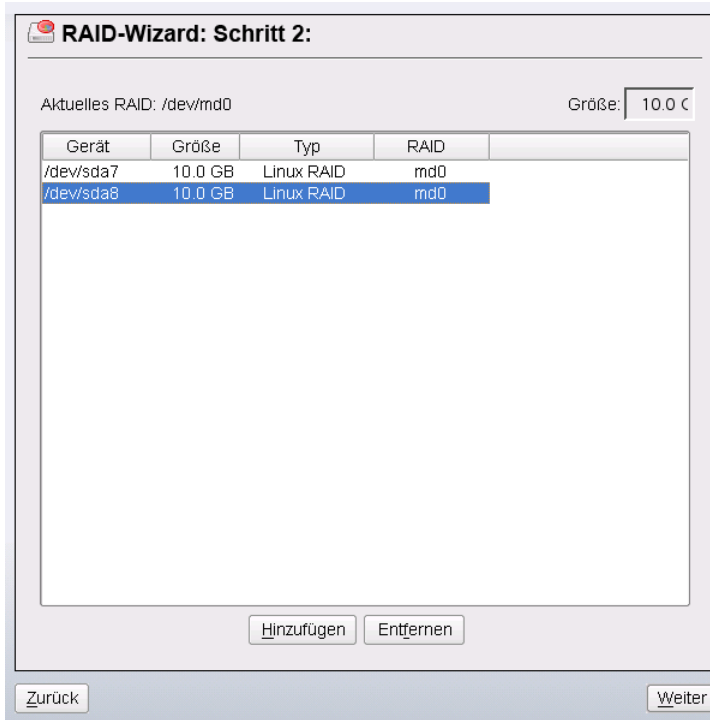
Abbildung 2.7 RAID-Partitionen
