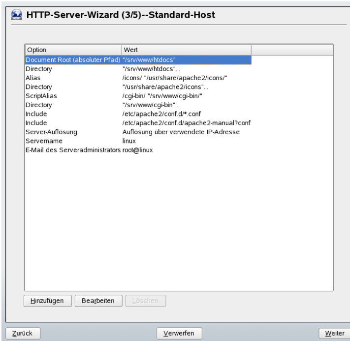
Abbildung 22.1 HTTP-Server-Wizard: Standardhost
