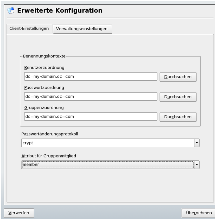
Abbildung 20.4 YaST: Erweiterte Konfiguration
