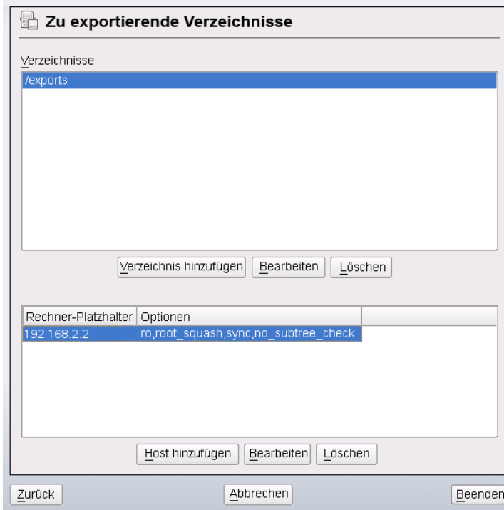
Abbildung 21.4 Exportieren von Verzeichnissen mit NFSv4
