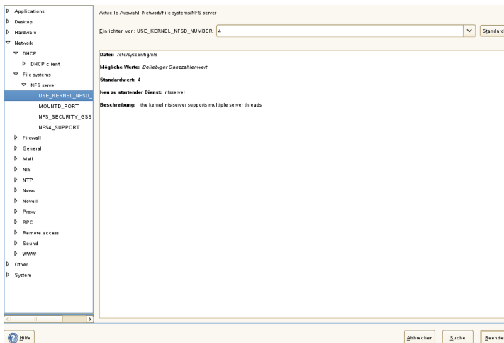
Abbildung 8.2 Systemkonfiguration mithilfe des sysconfig -Editors
