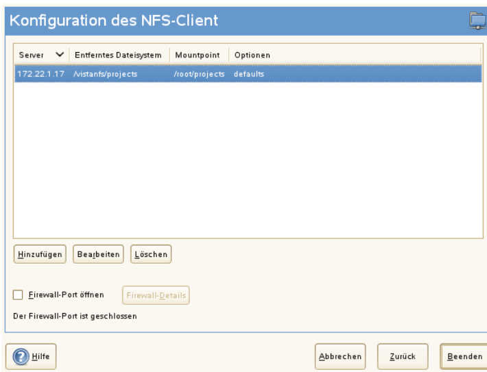
Abbildung 21.1 Konfiguration des NFS-Clients mit YaST
