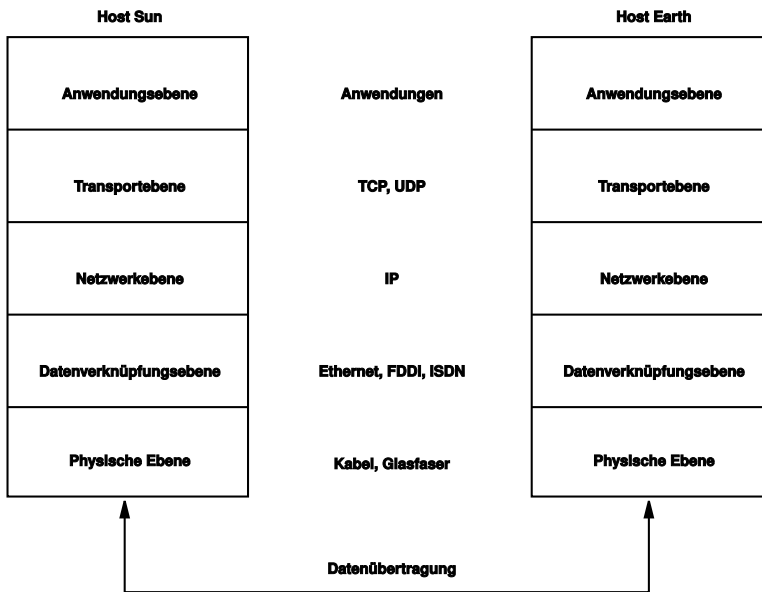
Abbildung 14.1 Vereinfachtes Schichtmodell für TCP/IP
