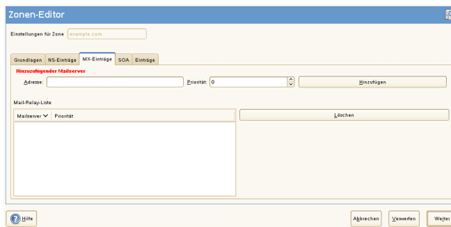
Abbildung 16.7 DNS-Server: Zonen-Editor (MX-Einträge)
