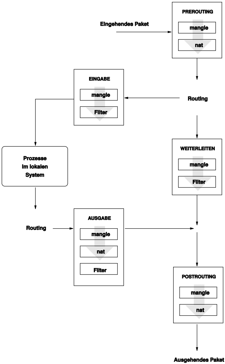
Abbildung 28.1 iptables: Die möglichen Wege eines Pakets
