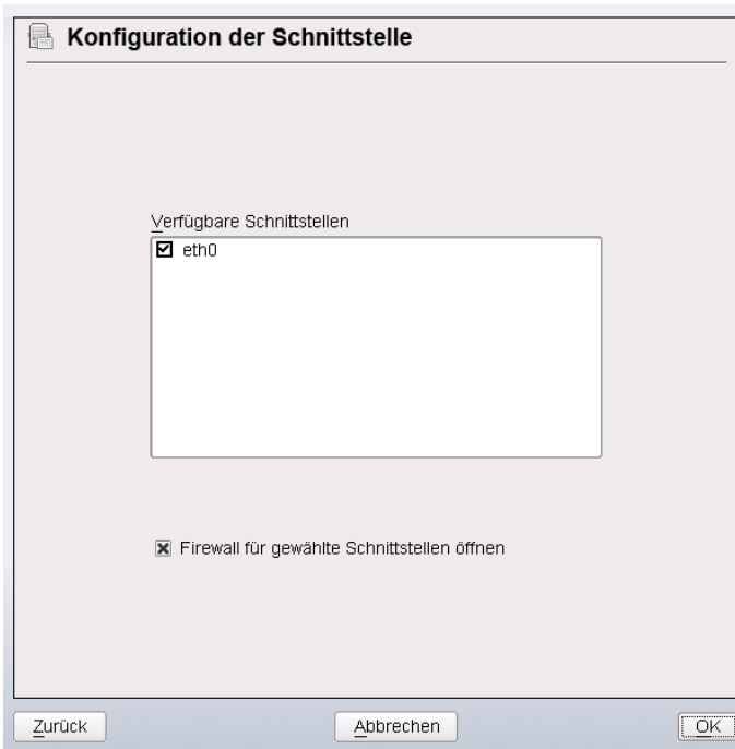
Abbildung 17.11 DHCP-Server: Netzwerkschnittstelle und Firewall
