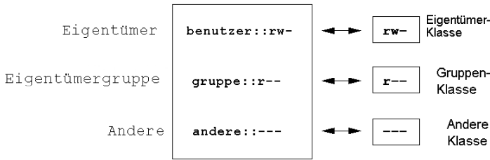
Abbildung 12.1 Minimale ACL: ACL-Einträge im Vergleich zu Berechtigungsbits
