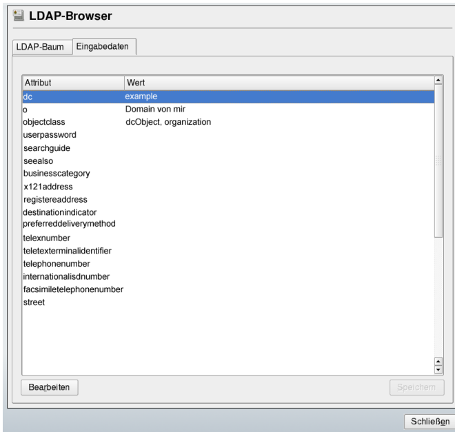
Abbildung 20.9 Navigieren in den Eingabedaten
