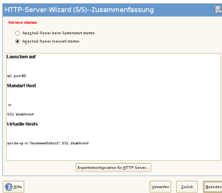
Abbildung 22.2 HTTP-Server-Wizard: Zusammenfassung
