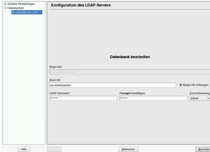
Abbildung 20.2 YaST-LDAP-Server-Konfiguration
