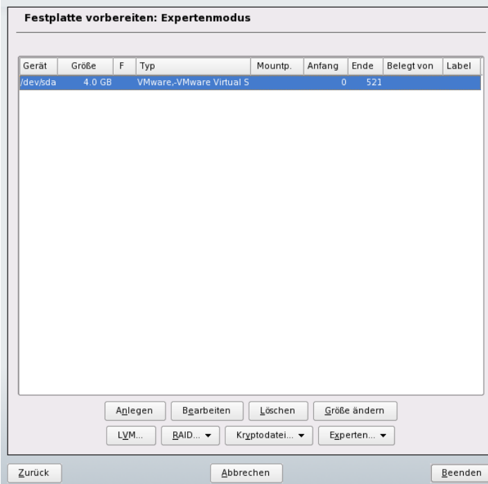
Abbildung 2.1 Die YaST-Partitionierung
