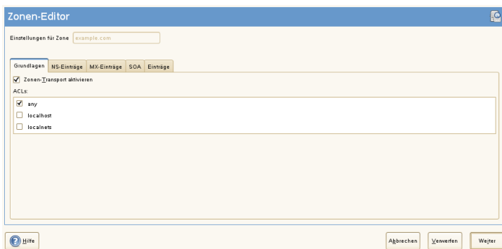
Abbildung 16.5 DNS-Server: Slave-Zonen-Editor
