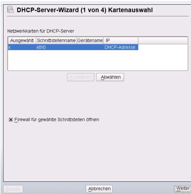
Abbildung 17.1 DHCP-Server: Kartenauswahl
