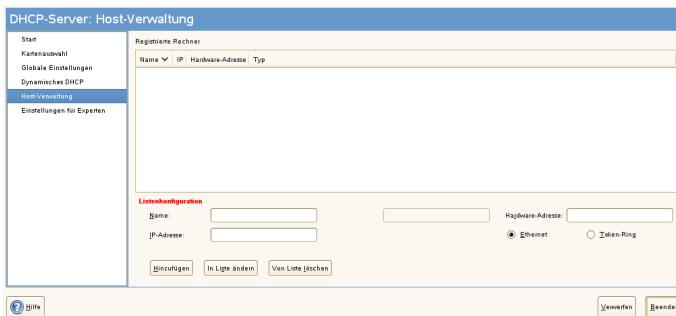
Abbildung 17.5 DHCP-Server: Host-Verwaltung
