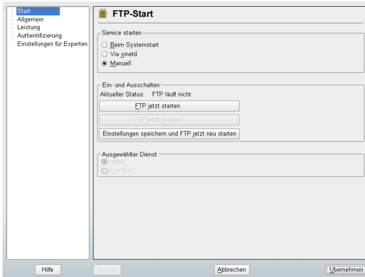
Abbildung 23.1 FTP-Serverkonfiguration - Start
