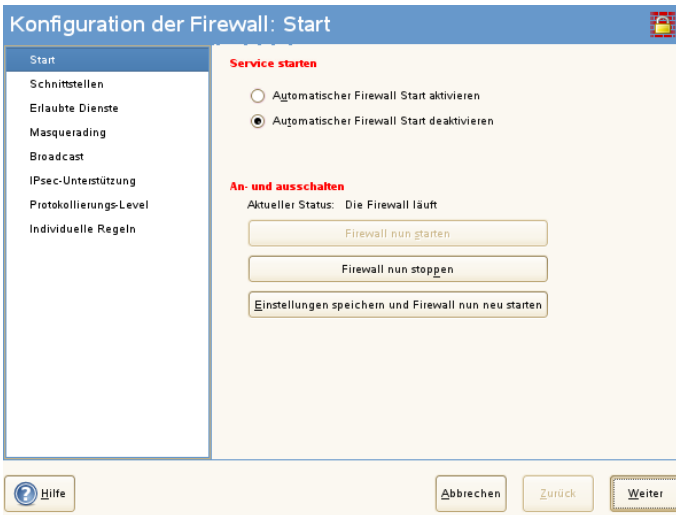
Abbildung 28.2 Die YaST-Firewall-Konfiguration
