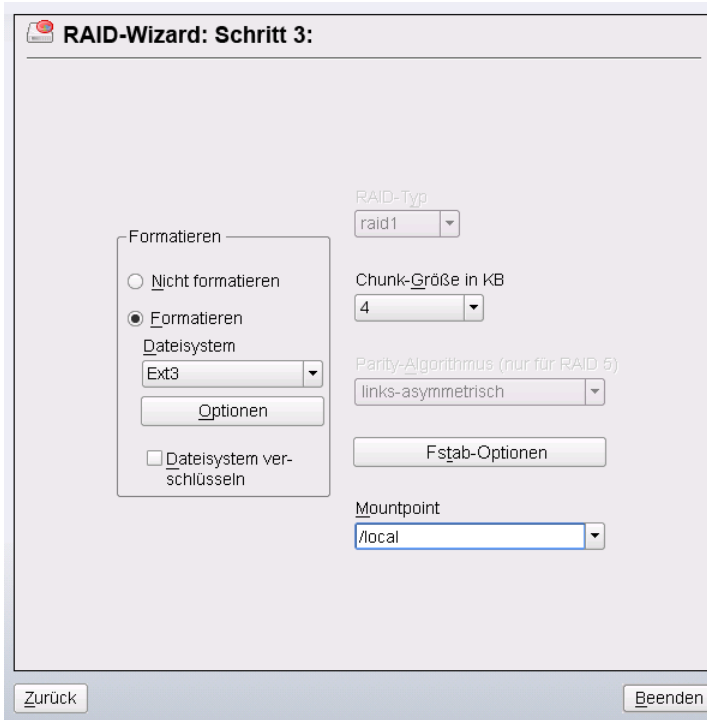
Abbildung 2.8 Dateisystemeinstellungen
