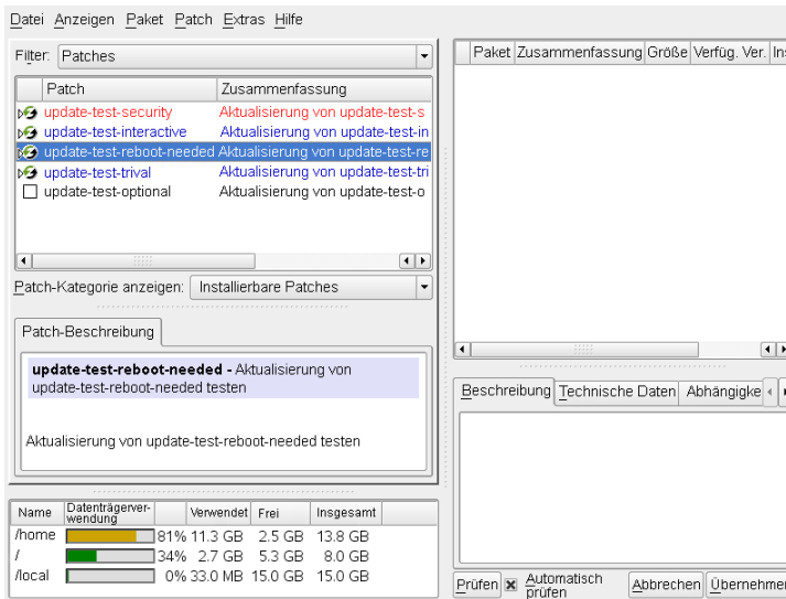
Abbildung 3.1 YaST-Online-Update
