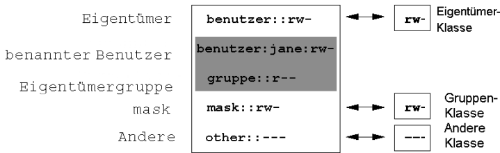
Abbildung 12.2 Erweiterte ACL: ACL-Einträge im Vergleich zu Berechtigungsbits
