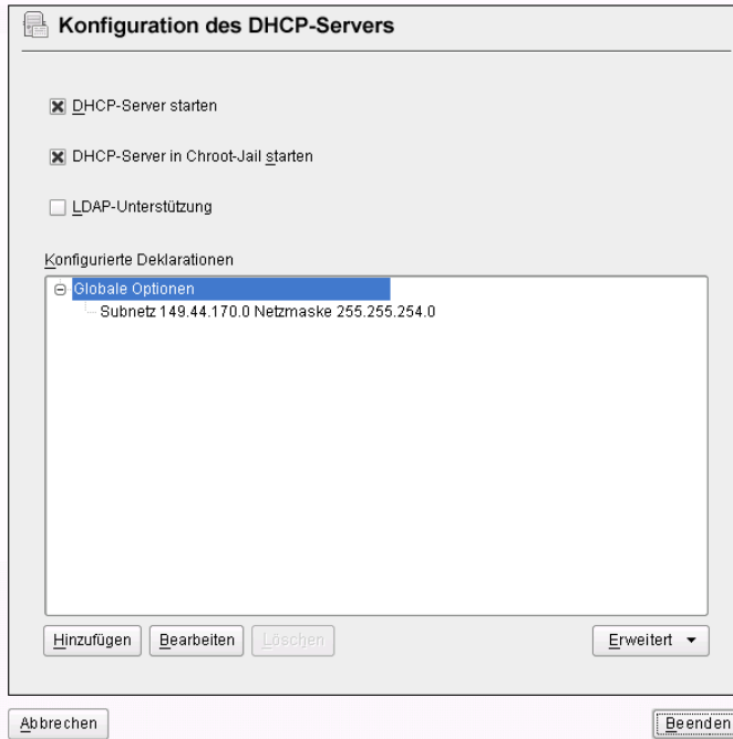
Abbildung 17.6 DHCP-Server: Chroot Jail und Deklarationen
