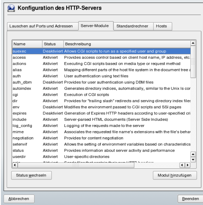
Abbildung 22.4 Konfiguration des HTTP-Servers: Server-Module
