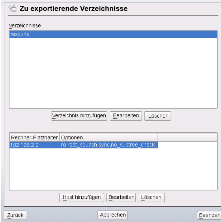
Abbildung 21.5 Exportieren von Verzeichnissen mit NFSv2 und v3
