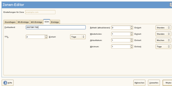
Abbildung 16.8 DNS-Server: Zonen-Editor (SOA)
