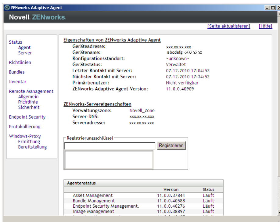
Abbildung 4-4 Eigenschaften von ZENworks Adaptive Agent
