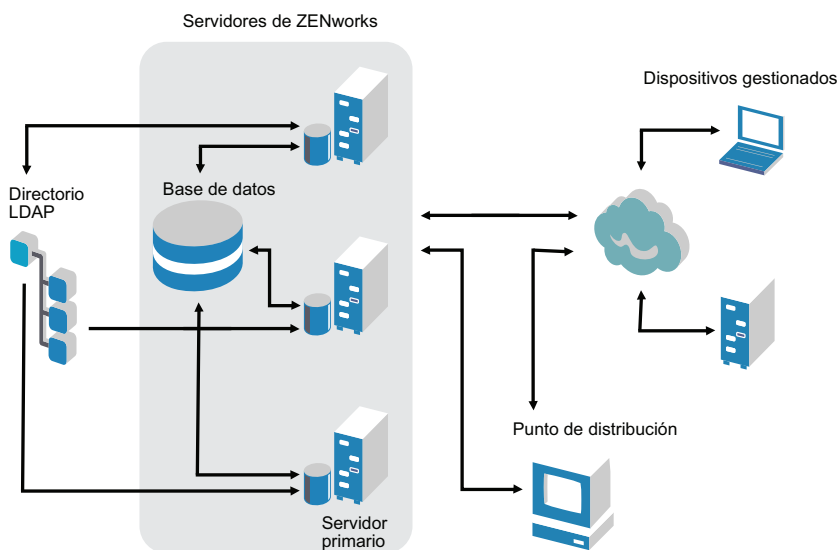
Figura 2-4 Arquitectura de ZENworks 10
