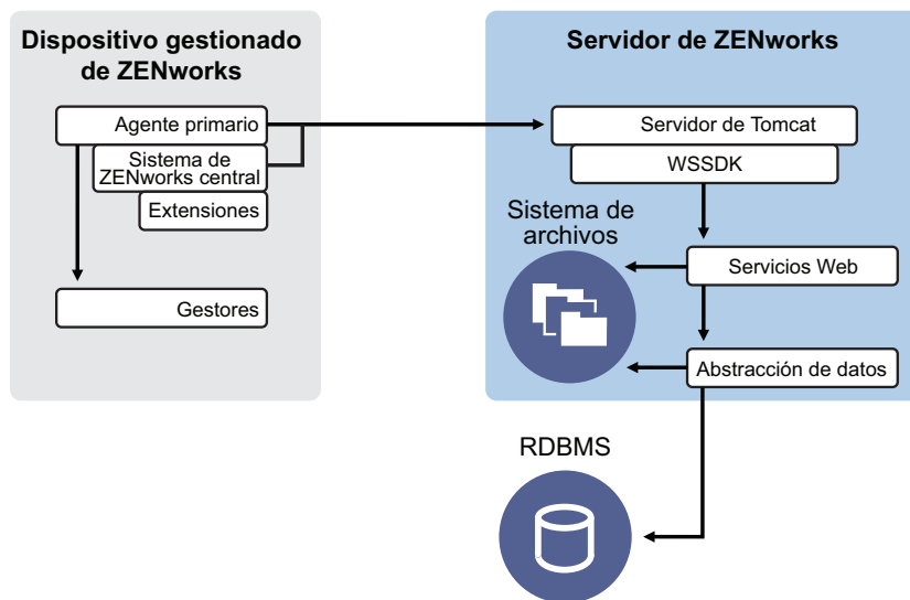
Figura 2-3 Arquitectura de clientes y servidores de ZENworks 10
