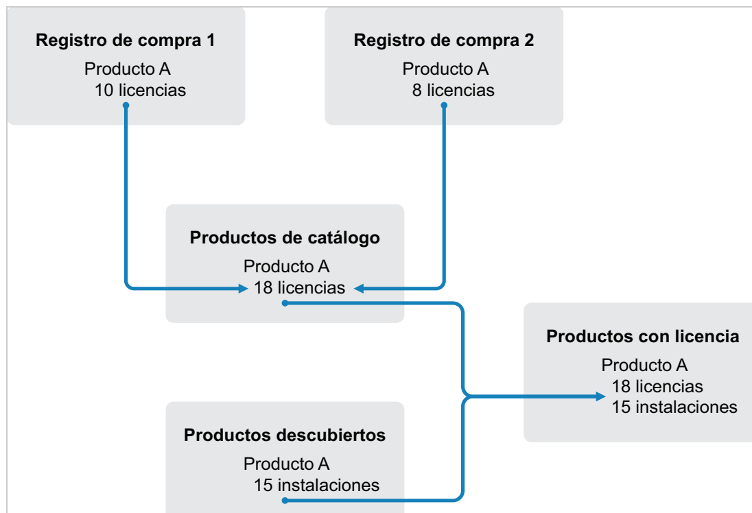
Figura 8-1 Componentes de conformidad de licencias
