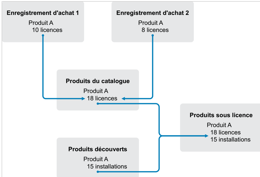
Figure 8-1 Composants de la conformité des licences
