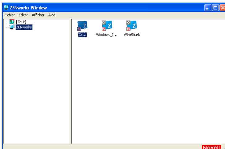
Figure 4-1 Fenêtre ZENworks
