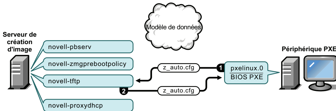
Figure 28-8 Phase 6 du processus des services de pré-lancement
