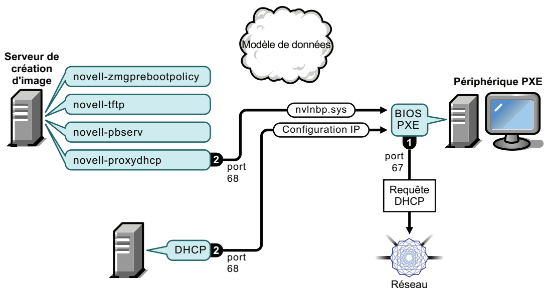
Figure 28-1 Configuration DHCP sur des serveurs séparés
