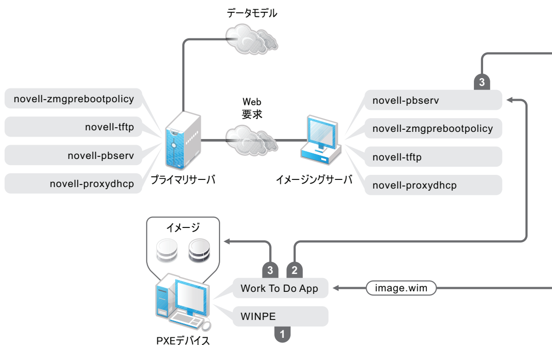
図 2-3 イメージングサテライト上のサードパーティイメージング用プレブートサービスプロセス
