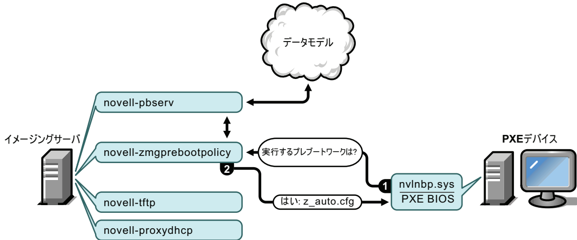
図 1-6 プレブートサービスプロセスのフェーズ4
