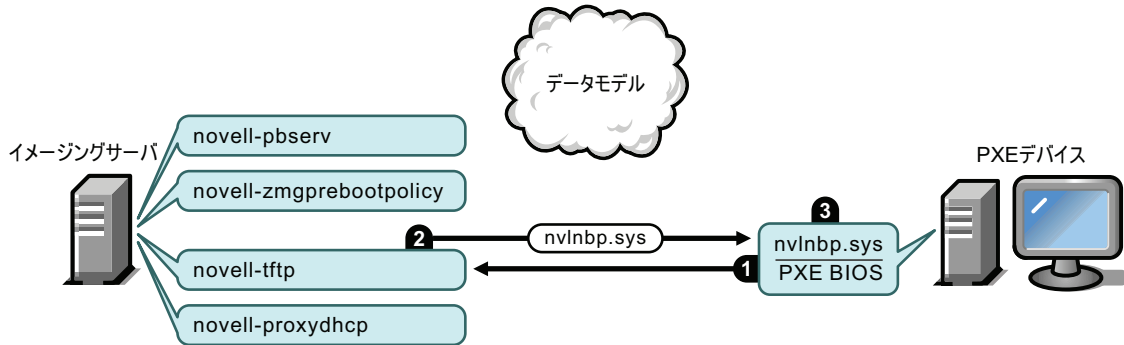
図 1-4 プレブートサービスプロセスのフェーズ2
