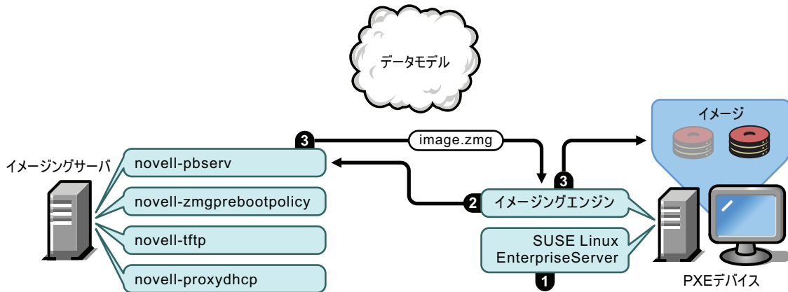
図 1-10 ZENworks Imaging のプレブートサービスプロセスのフェーズ 8
