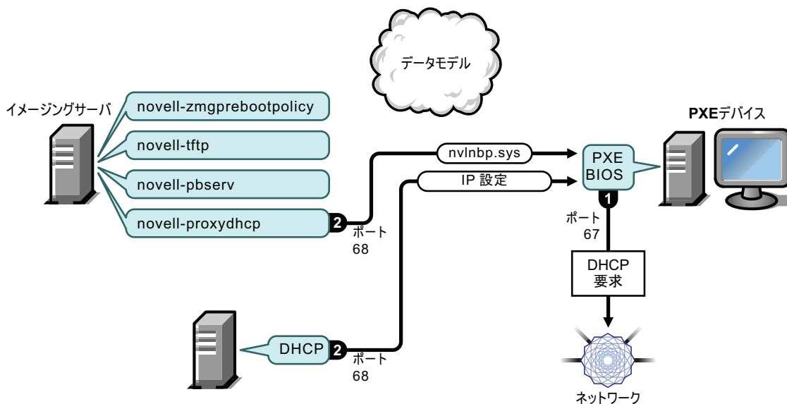
図 1-1 異なるサーバにおける DHCP 設定
