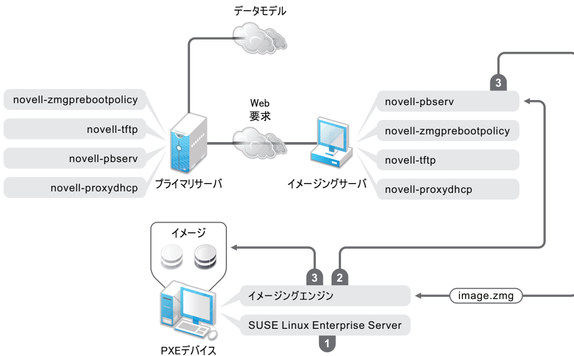
図 2-2 イメージングサテライト上の ZENworks Imaging 用プレブートサービスプロセス
