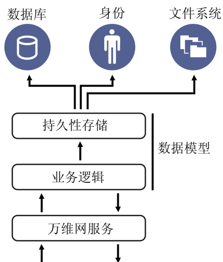
图 2-2 ZENworks 10 三层结构
