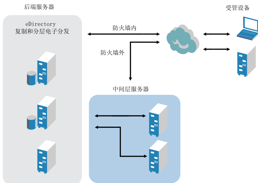
图 2-1 ZENworks 桌面管理结构
