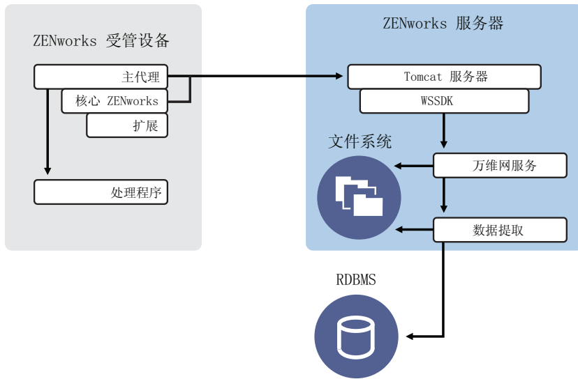
图 2-3 ZENworks 10 客户端 - 服务器结构
