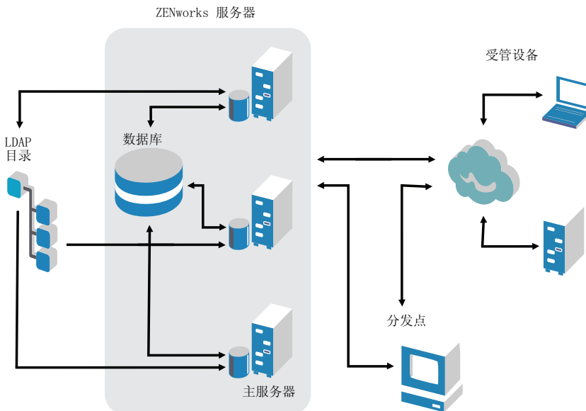
图 2-4 ZENworks 10 结构
