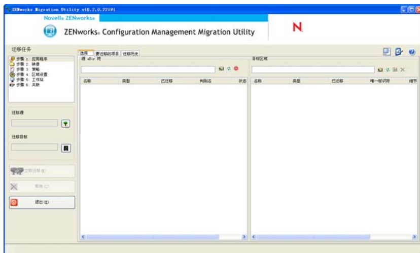
图 C-1 ZENworks 迁移实用程序
