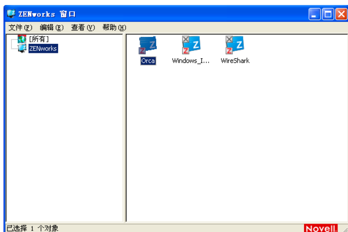
图 7-1 ZENworks 窗口
