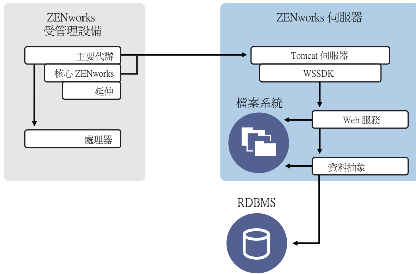
圖 2-3 ZENworks 10 用戶端- 伺服器結構
