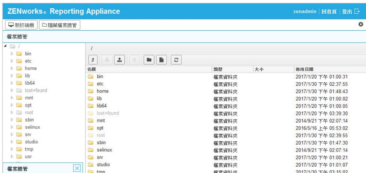
圖 6-5 檔案總管
