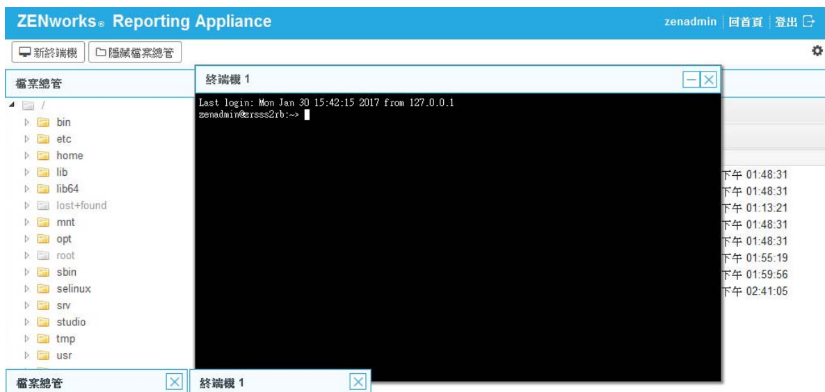
圖 6-4 終端機
