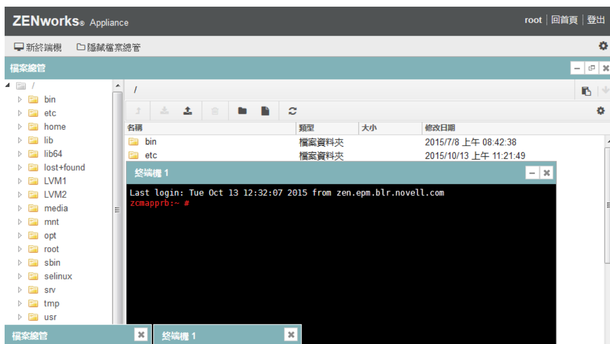
圖 6-4 終端機
