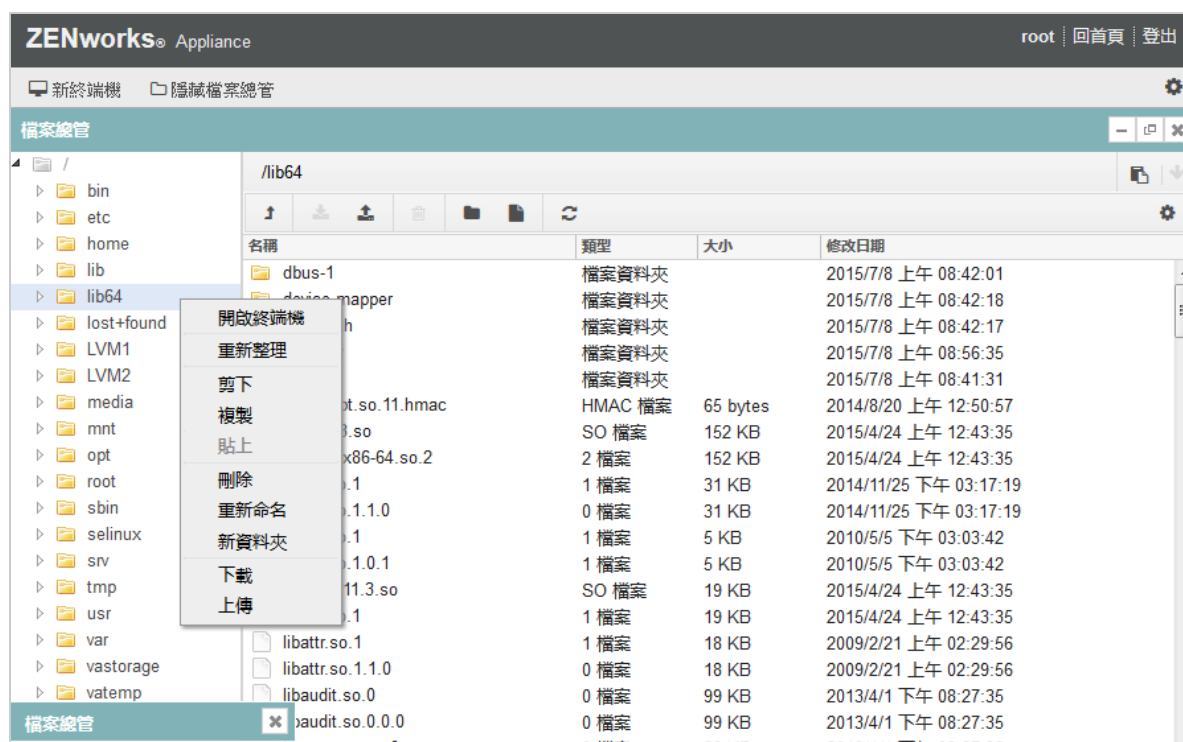
圖 6-5 檔案總管
